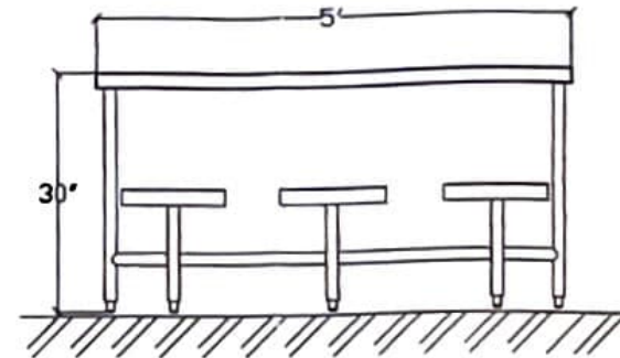
ELEVATION A-A
